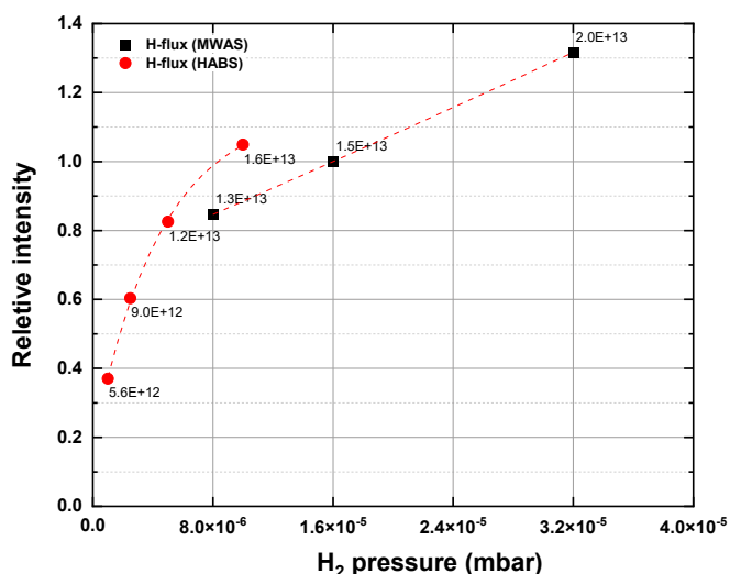
Figuur 4. Kalibratie van de H-atoomflux voor de HABS- en de MWAS-bron als functie van de H_2 -inlaatdruk.
