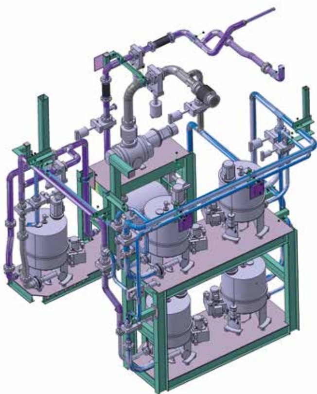
Figuur 7. 3D-model van de CRS-pompinstallatie; rechts: vier scrollpompen; links: één Roots-pomp, een buffertank en één scrollpomp.
