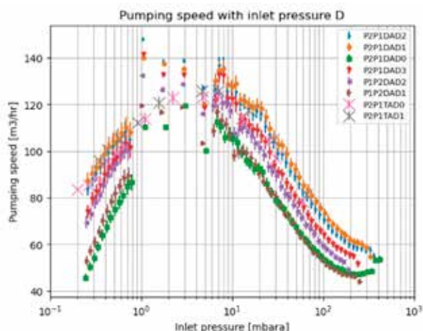
Figuur 5. Deuteriumtest van twee Eumeca 150 m³/uur scrollpompen in serie. Rechts de legenda voor de verschillende tests. De eerste test, weergegeven in blauw (P2P1DAD2), betekent bijvoorbeeld dat pomp 2 als eerste in serie was geschakeld en ondersteund werd door pomp 1. Deze test was een vacuümtest waarbij de pomp werd leeggemakt tot omgevingsdruk met deuterium, en was de tweede test met deze configuratie.
