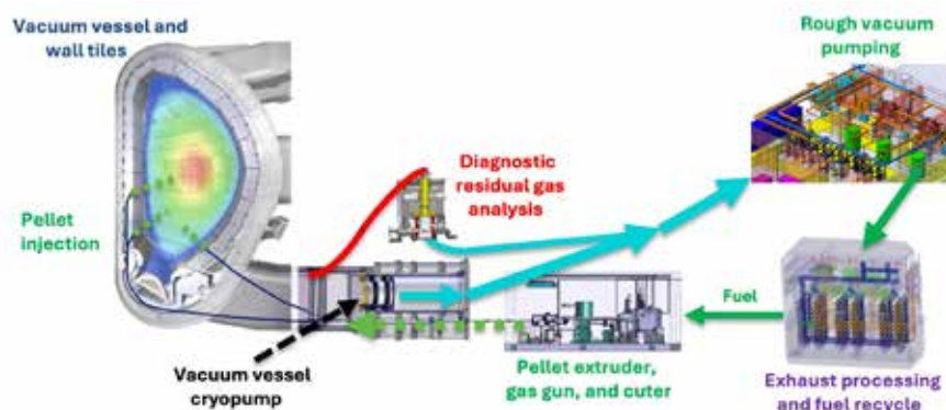
Figuur 2. De ITER-brandstofcyclus.
