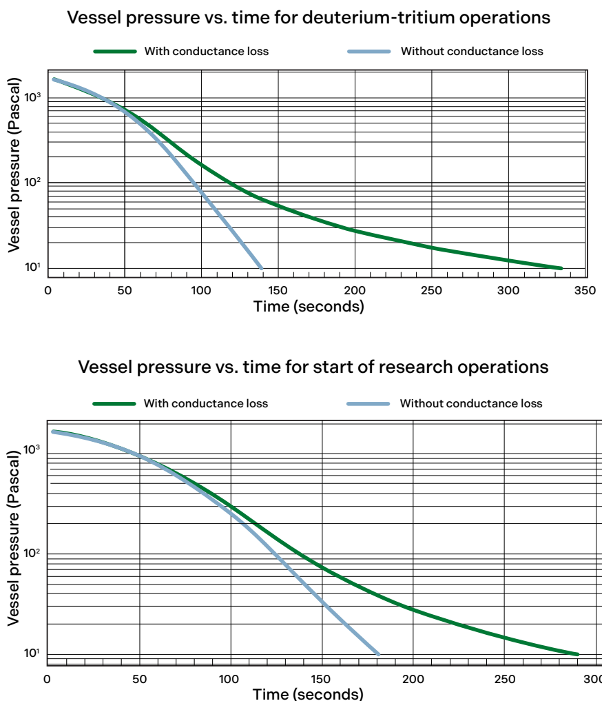
Figuur 8. Evacuatie van een TCP van 1.754 Pa naar 10 Pa.
