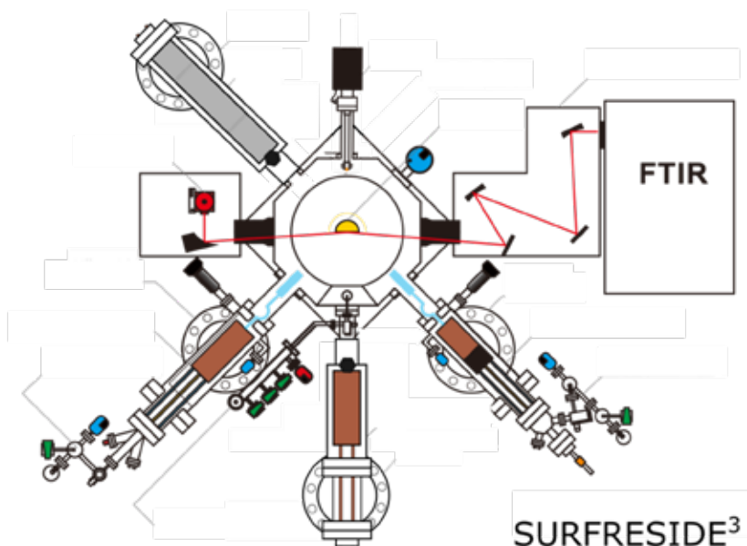
Figuur 3. Schematisch bovenaanzicht van SURFRESIDE.
