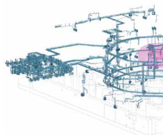
Figuur 1. Vacuümscope van de US binnen het ITER-project, met de RPS links in blauw omcirkeld.
