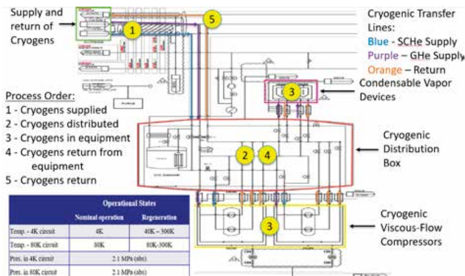
Figuur 3. Stroomschema van cryogene vloeistoffen in het cryogene systeem. Zie de tekst voor toelichting op de nummers.
