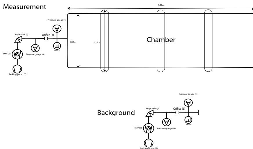
Figuur 2. Schematische weergave van de meetprocedure. Eerst wordt een achtergrondmeting uitgevoerd met alleen de meetopstelling (Background), zonder het prototype. Vervolgens wordt dezelfde meting herhaald met het prototype geïnstalleerd (Measurement), zodat de bijdrage van het prototype aan de gemeten vacuümeigenschappen kan worden bepaald.
