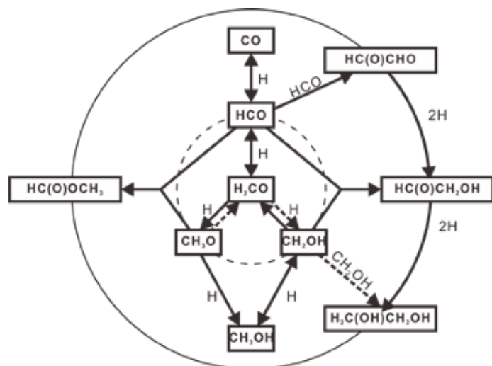
Figuur 10. Interstellaire CO-ijschemie aangedreven door H-atomen op het oppervlak van interstellaire stofdeeltjes. (Bron: [18])
