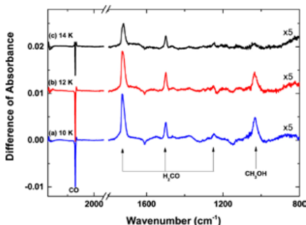
Figuur 8. IR-verschilspectra verkregen na blootstelling van CO-ijs aan H-atomen bij (a) 10 K, (b) 12 K, en (c) 14 K. Negatieve en positieve signalen weerspiegelen netto verbruik en vorming, respectievelijk. (Bron: [16])
