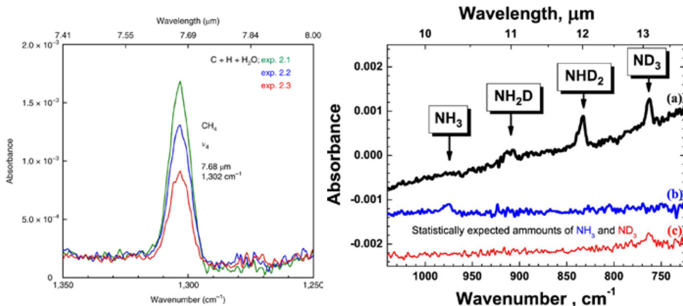
Figuur 7. IR-spectra van hydrogeneringsroutes. (Bron: [12-13])
