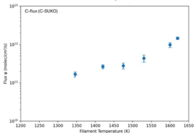
Figuur 5. Kalibratie van de C-atoomflux voor de C-SUKO-bron als functie van de sublimatietemperatuur van het filament.
