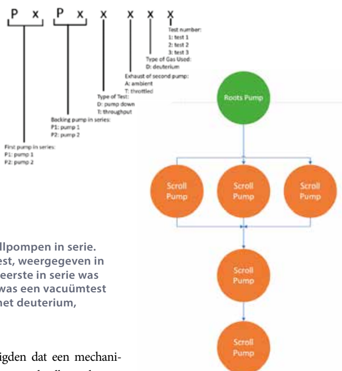
Figuur 6. Processtroomschema van de hoofdconfiguratie van de CRS-pomptreinen (exclusief bypasses).
