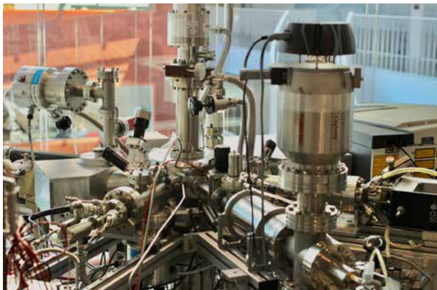
Figuur 2. Experimentele opstelling SURFRESIDE in LfA. (Foto: Franciele Kruczkiewicz)
