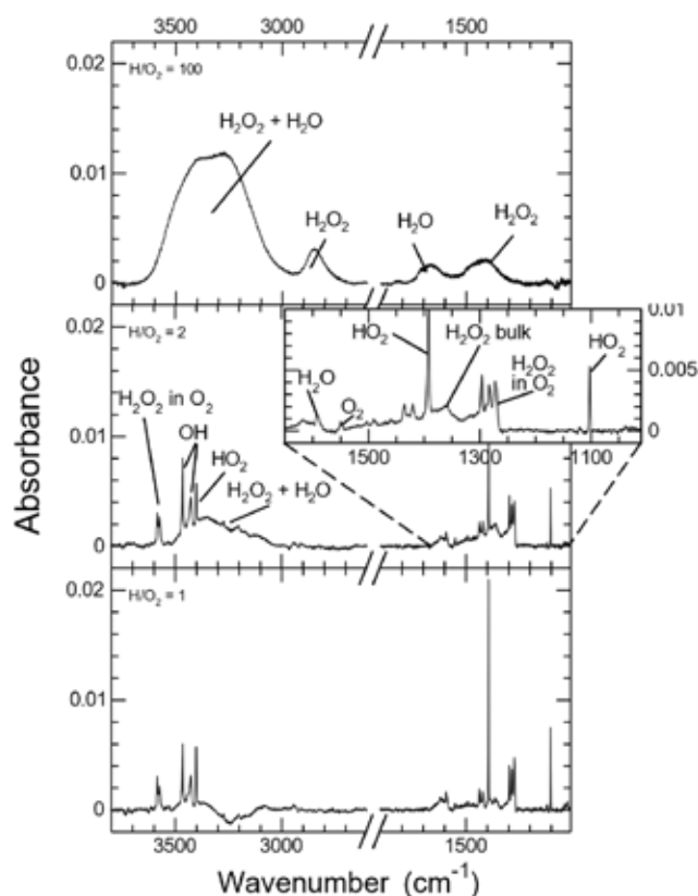
Figuur 6. IR-spectra van experimenten met co-depositie van H en O 2 bij 20 K, met H 2 O 2 -verhoudingen van respectievelijk 100, 2 en 1 (van boven naar beneden). (Bron: [10])
